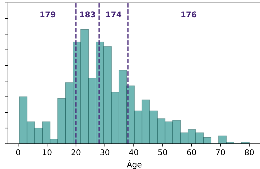
(b) Classes d'effectifs égaux (qcut)
