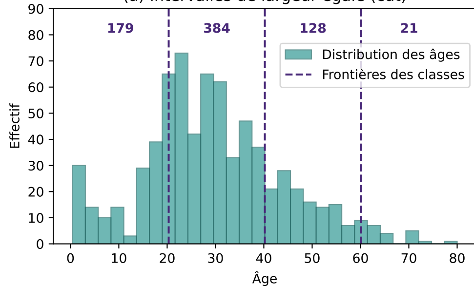
(a) Intervalles de largeur égale (cut)
